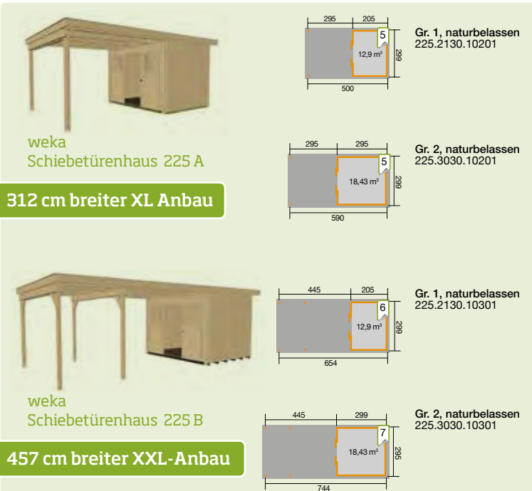
weka Schiebetürhaus 225 Gr. 1 · 225.2 130.10201
