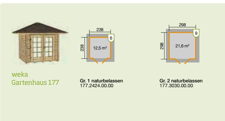
weka Gartenhaus 177 Gr. 1 · Abb. 177.2424.00.00 · mit Zubehör Dachschindeln (gegen Aufpreis)
