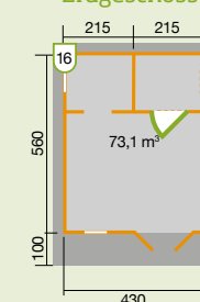
Erdgeschoss
