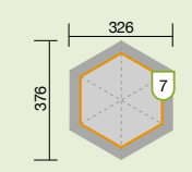
Gr. 1 ohne Dachschindeln 656.3030.00.00
