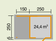
Designhaus „wekaLine“ 413 A
