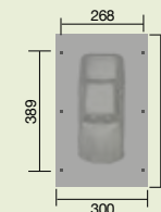
weka Carport 606 Gr. 1 max. Schneelast: si=0,68 kN/m 2
