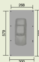
weka Carport 606 A Gr. 2 max. Schneelast: si=0,85 kN/m 2 inkl. Leimholzbogen
