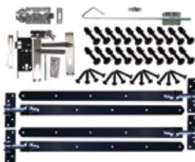
39.1025 Ensemble complet de ferrures noires et serrure à cylindre en inox Pour porte renforcée double en mélèze/douglas
