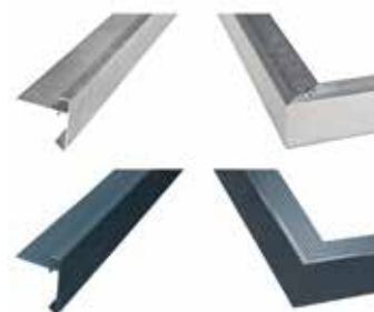
40.1114 250x4.5x4.5 cm Tout droit 40.1115 50x4.5x4.5 cm angle extérieur 40.1114Z 250x4.5x4.5 cm anthracite, tout droit 40.1115Z 50x4.5x4.5 cm angle extérieur anthracite
